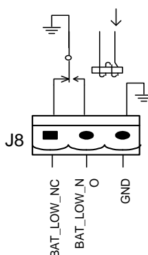
Рисунок 17. Сухой контакт сигнала о низком заряде АКБ
