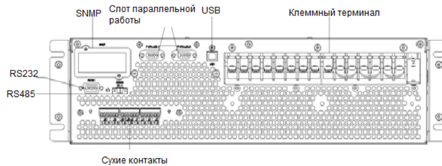
Рисунок 1. (б) Внешний вид ИБП 10-15 КВА (вид сзади)
